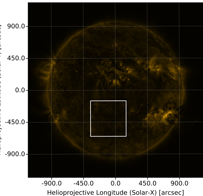
AIA 171 Å 2011-06-07 06:33:02
