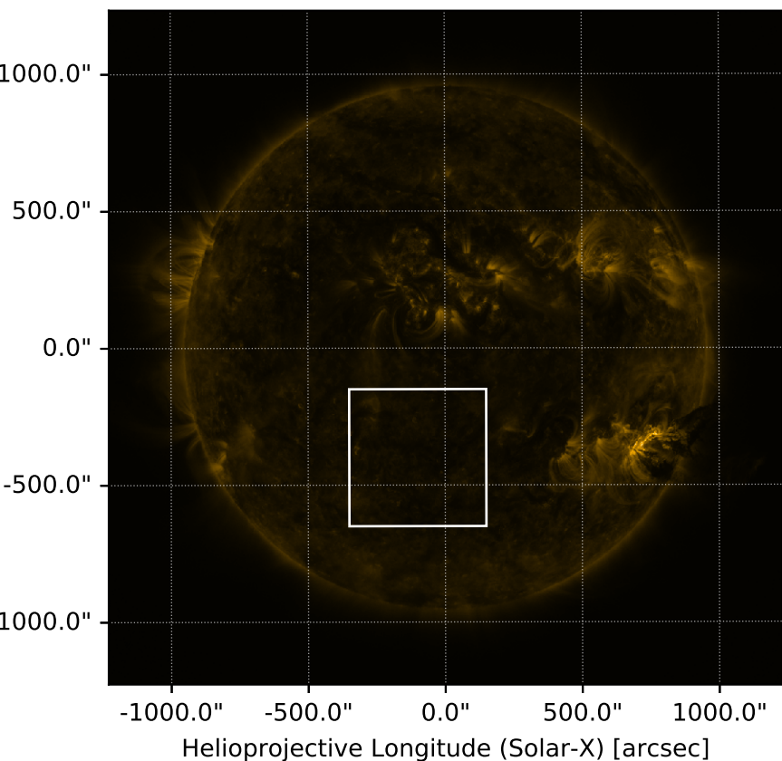
AIA 171 Å 2011-06-07 06:33:02
